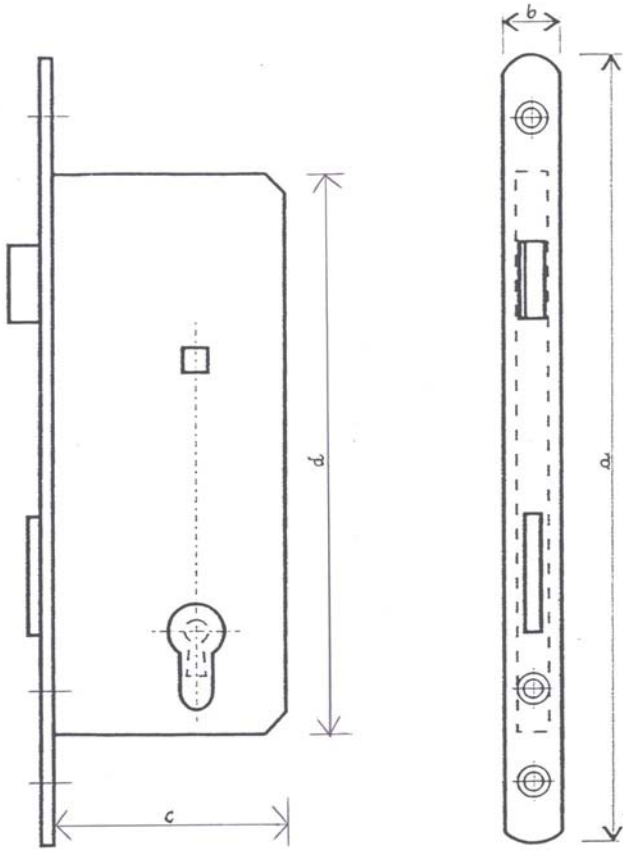
Rys. 1 Zamek drzwiowy wpuszczany
