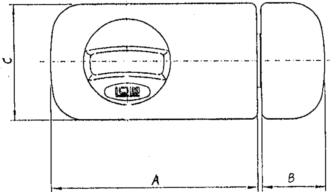
Rys. 2 Zamek drzwiowy nakładany
