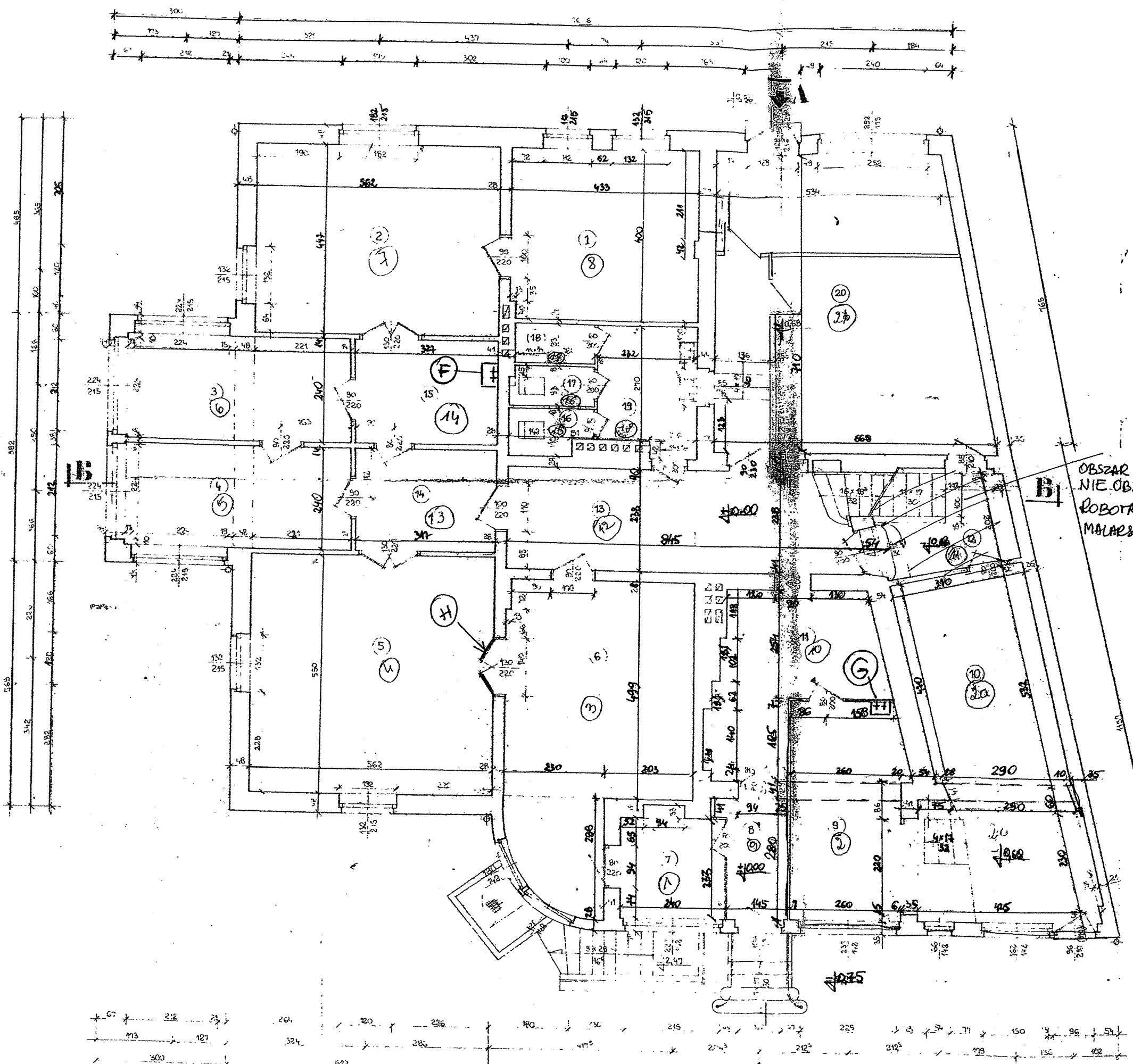
RZUT PARTERU
