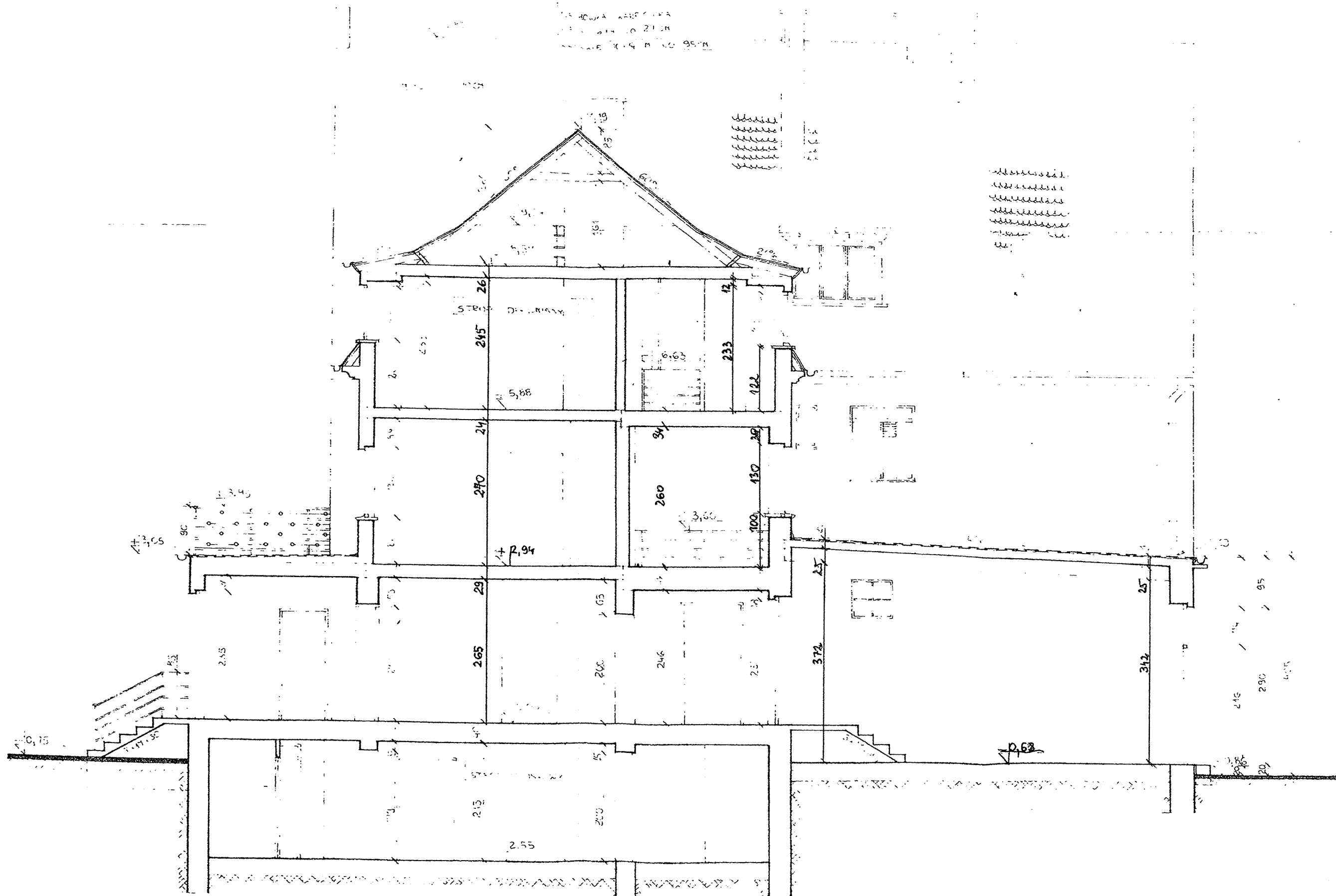
PRZEKRÓJ A-A 1:50
