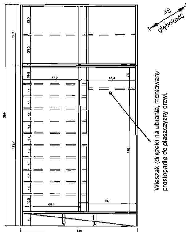
② - Szafa biurowo-ubraniowa (drzwi rozsuwane) 140x45x266 cm - 1 szt. półki w szafie wsparte na wspornikach metalowych z możliwością regulacji +/- 64 mm
