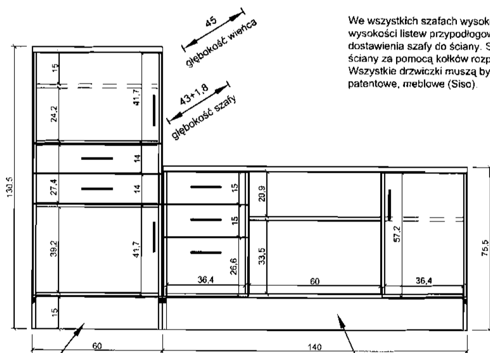
④ - Szafa przystawka do biurka 140x45x75 cm - 1szt.
