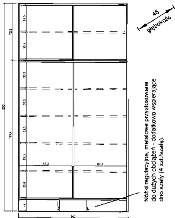
① - Szafa biurowa (drzwi rozsuwane) 140x45x266 cm - 2 szt. półki w szafie wsparte na wspornikach metalowych z możliwością regulacji +/- 64 mm
