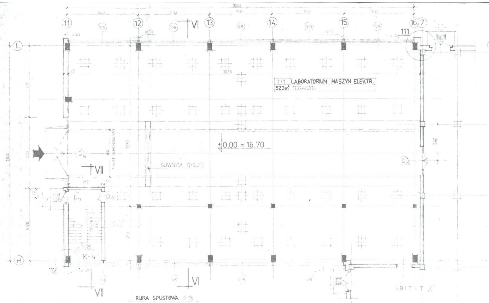
Rzut przyziemia – obiekt B
