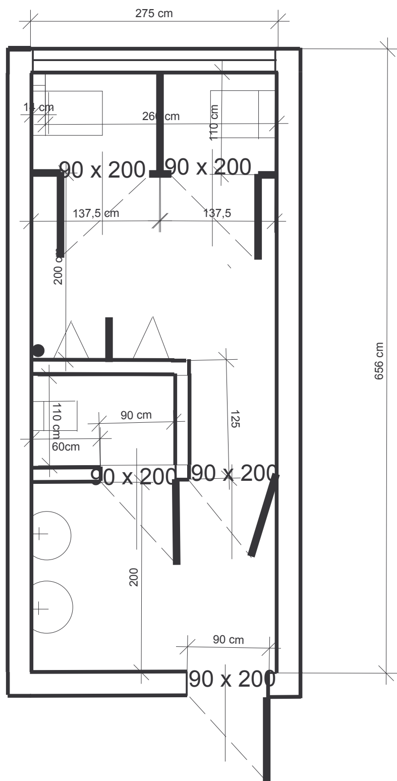
rzut typowej kondygnacji
