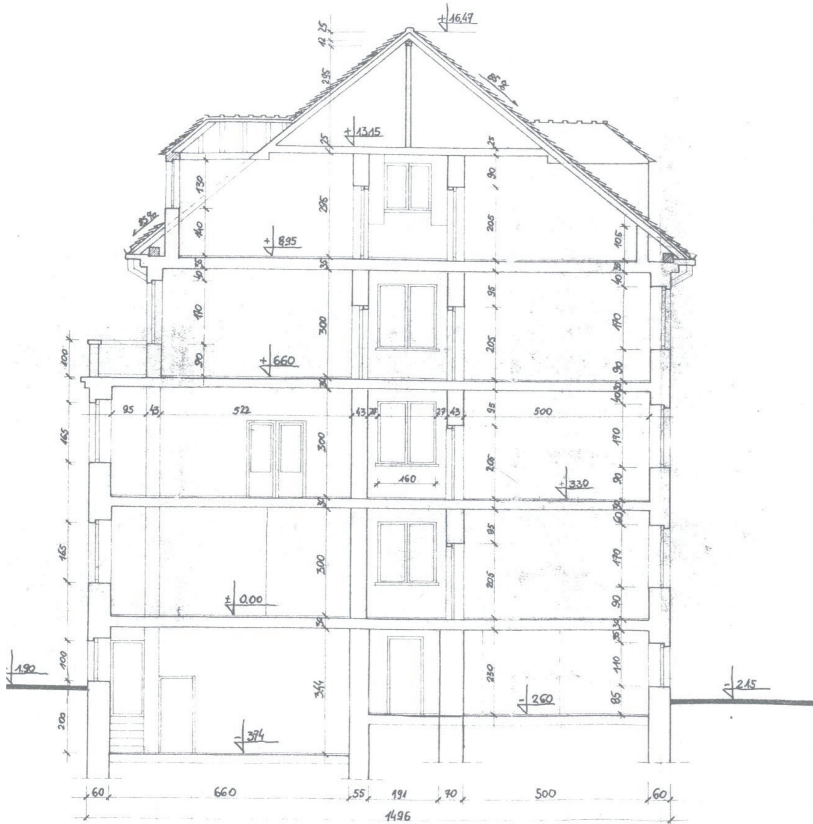
PRZEKRÓJ A-A 1:100
