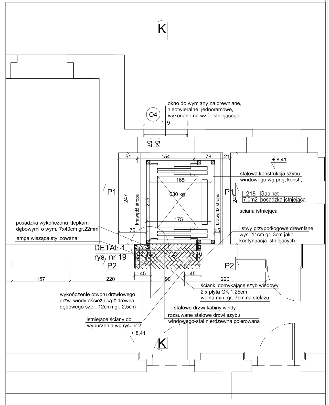
WINDA - RZUT II PIĘTRA
