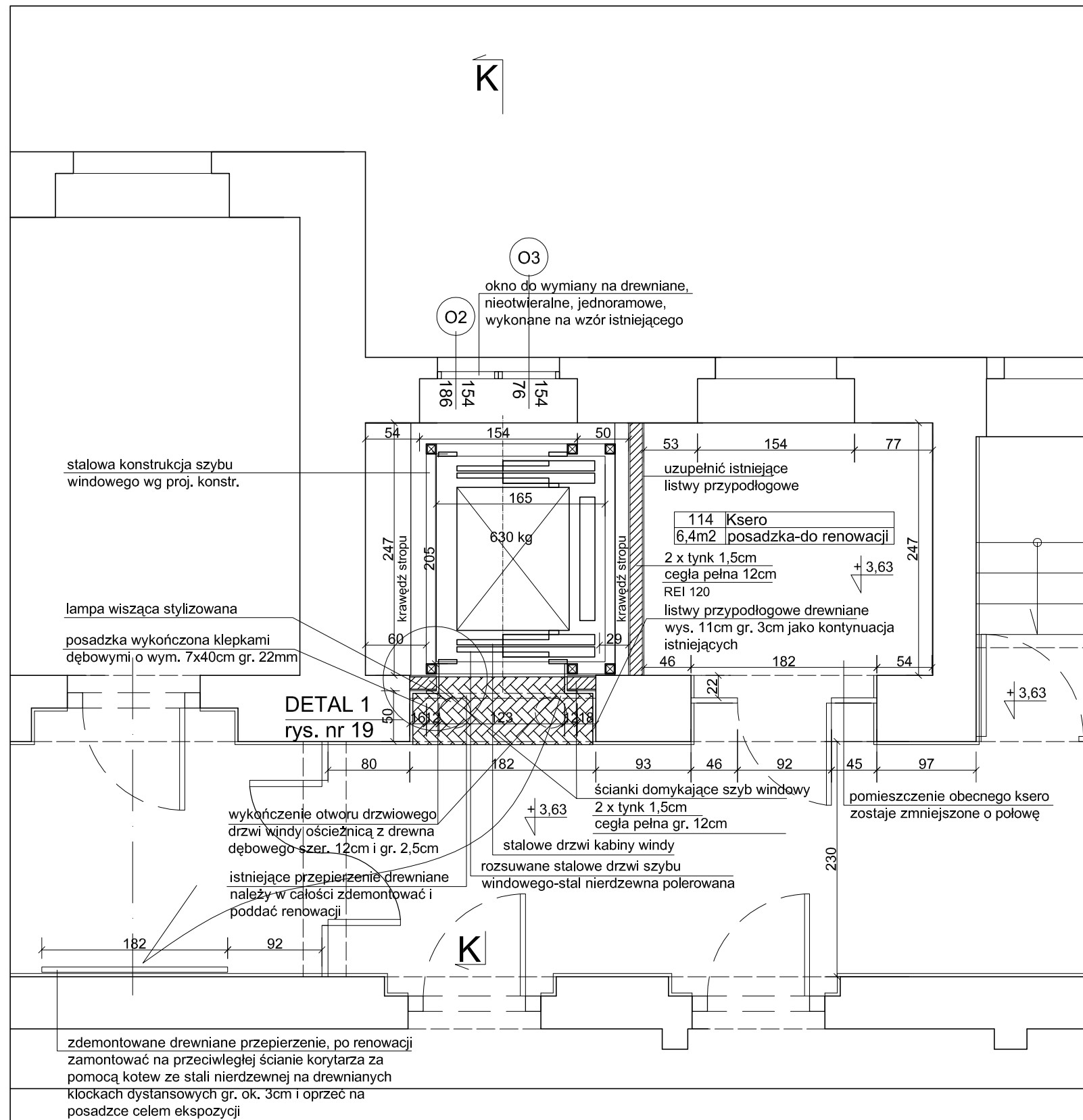
WINDA - RZUT I PIĘTRA
