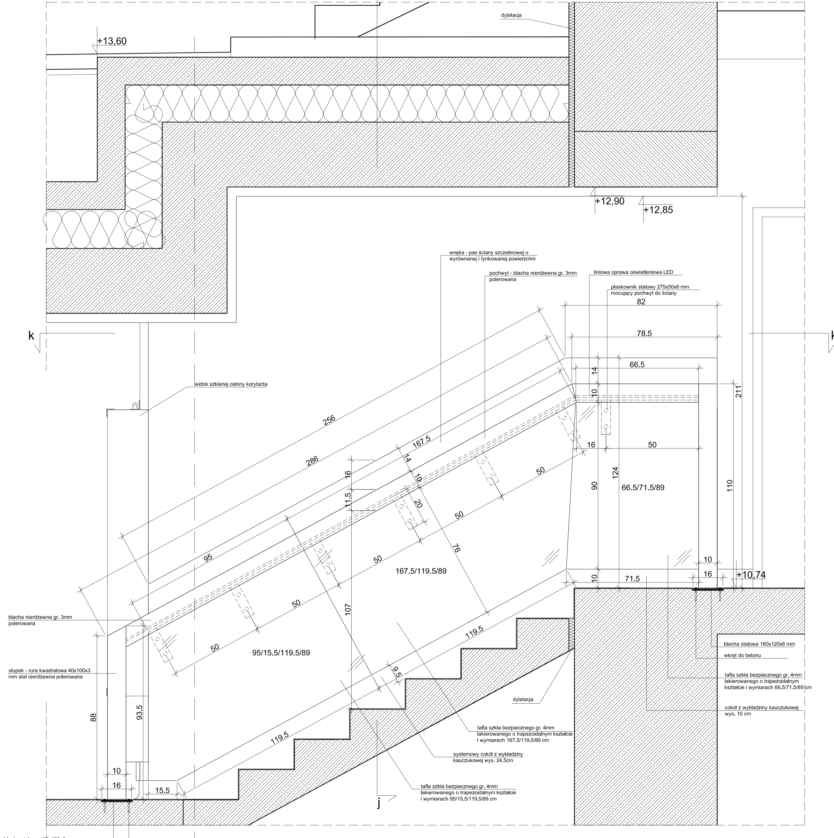
PRZEKRÓJ h - h
