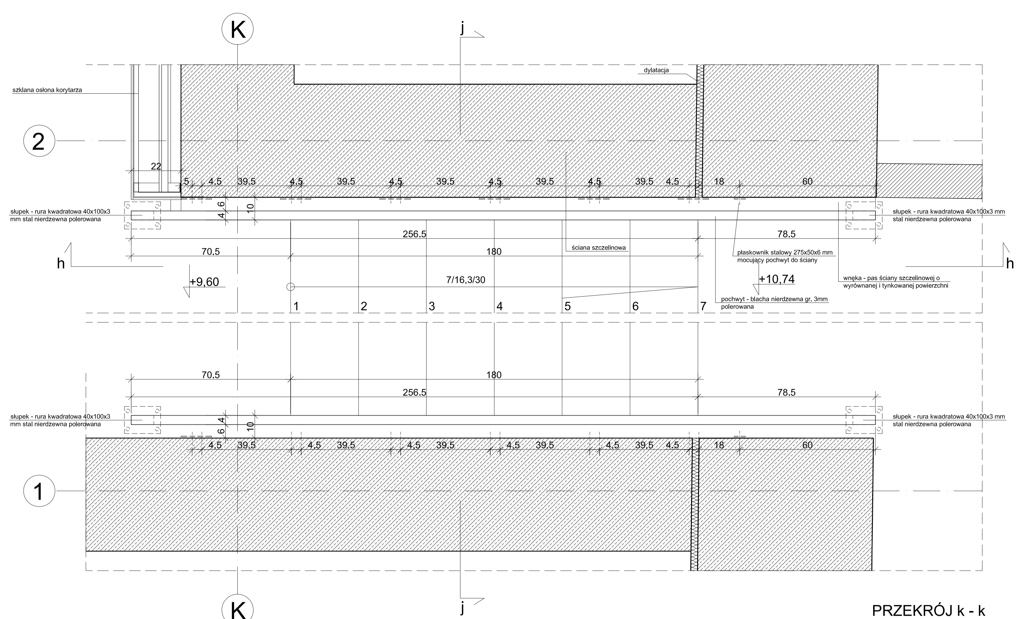
PRZEKRÓJ k - k
