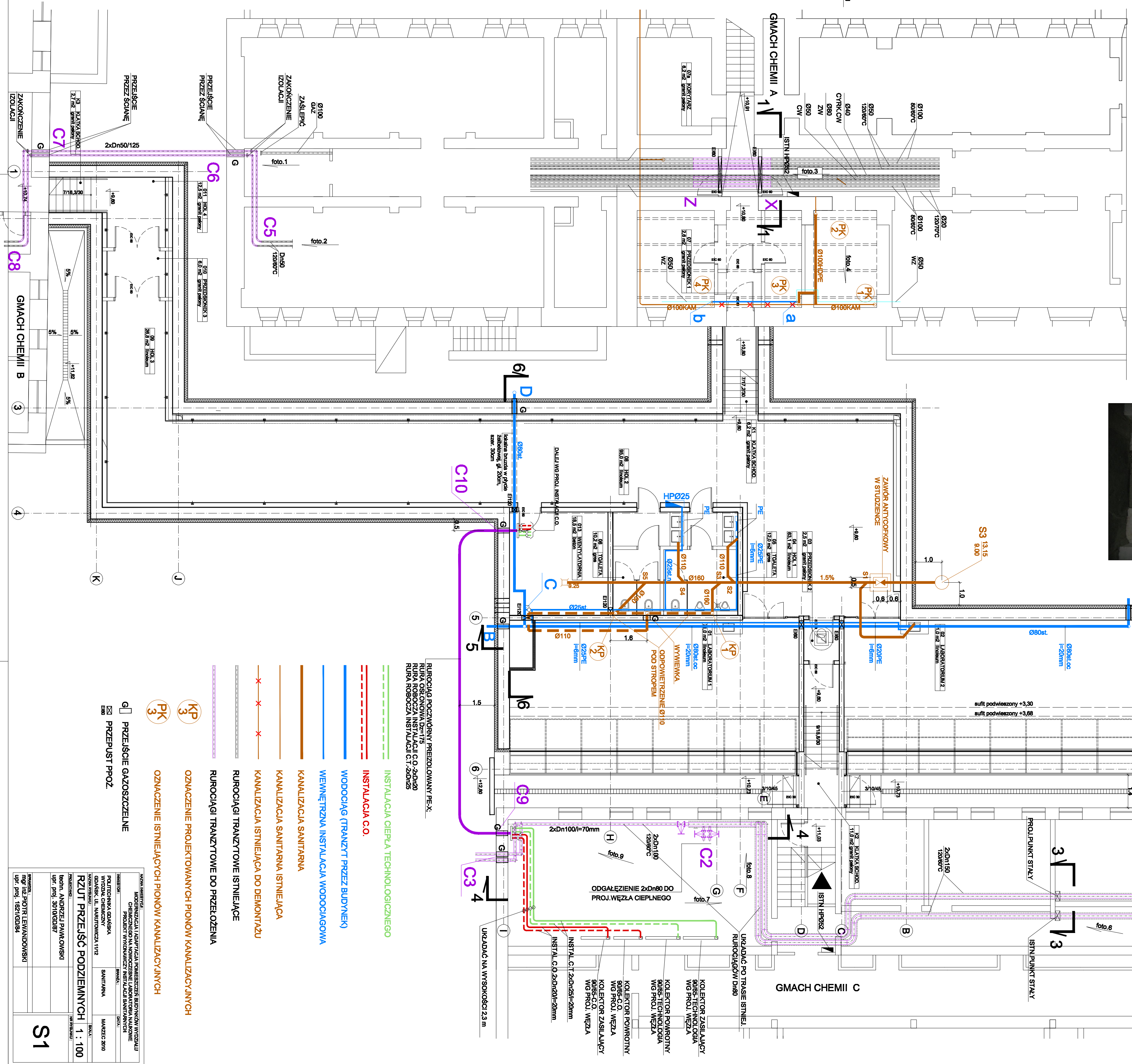
foto. 7 TRASA UKŁADANIA PROJEKTOWANEJ SIECI 2xØdn190
