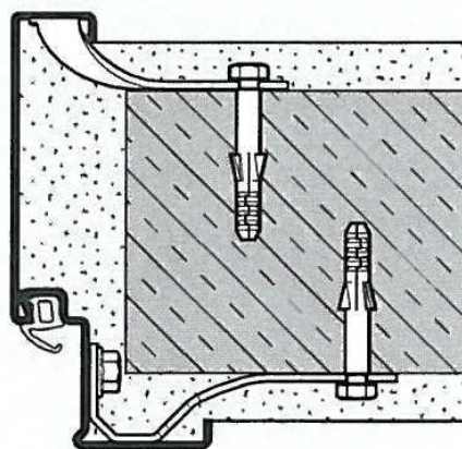
Ościeżnica obejmująca Montaż za pomocą kotew pod kołki rozporowe do zamurowania
