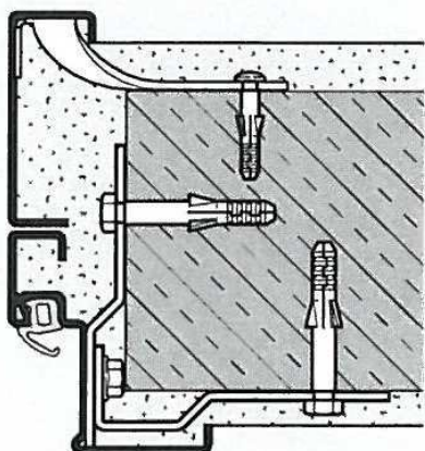
Ościeżnica kątowna z ościeżnicą uzupełniającą Montaż za pomocą kotew pod kołki rozporowe do zamurowania
