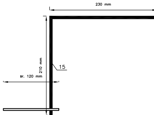
WIDOK Z BOKU MOCOWANIE SOND
