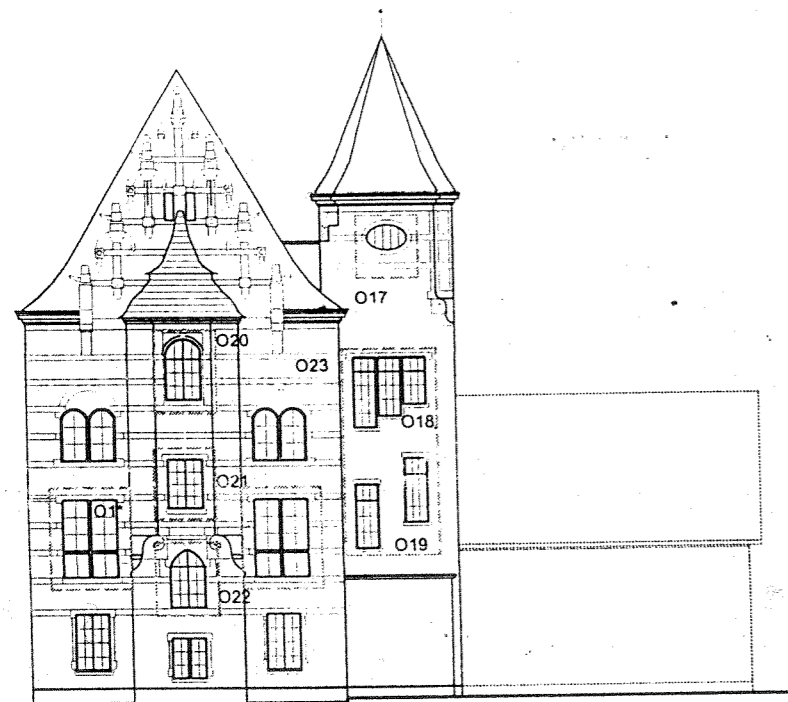
ELEWACJA D1 - PÓŁNOCNO-WSCHODNIA
