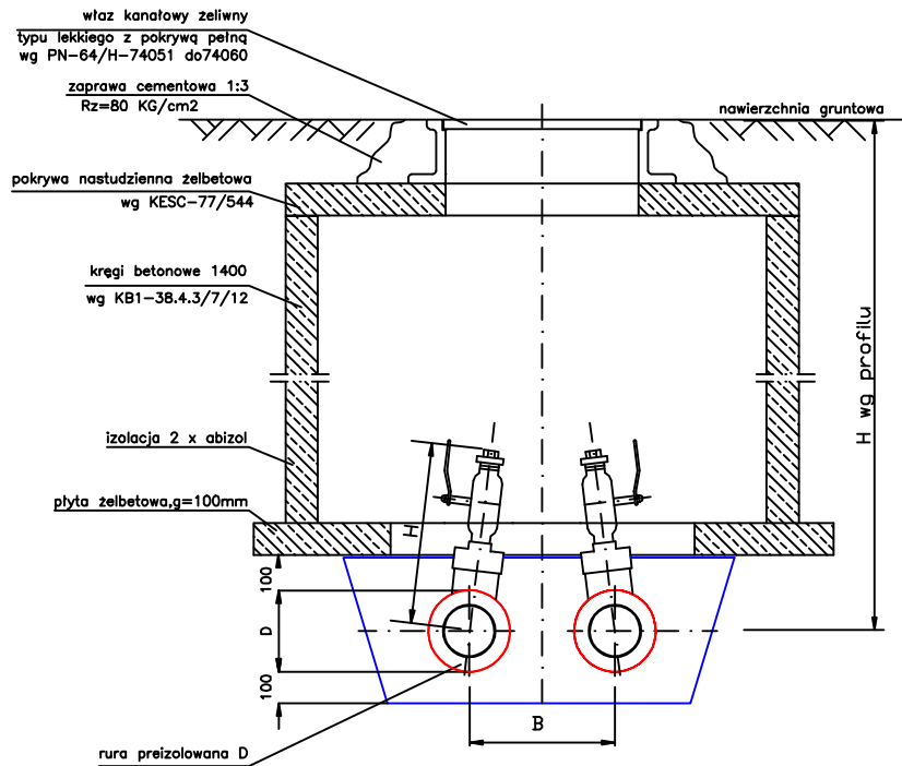
Przekrój A-A
