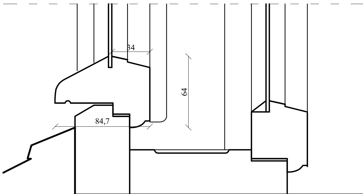
PRZEKRÓJ PIONOWY
