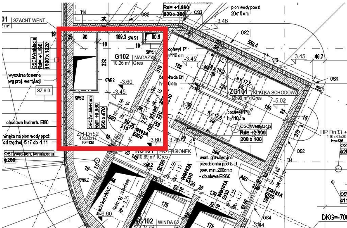
-fragment oznaczony czerwoną obwiednią gdzie ściany g-k mają wysokość 270 cm
