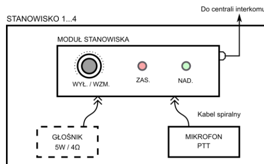
Rys. 2. Schemat blokowy stanowiska
