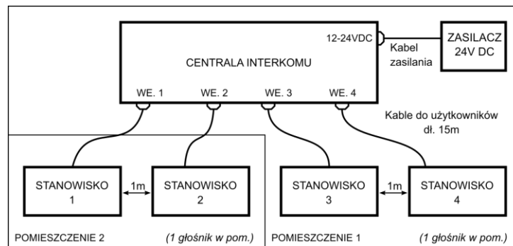
Rys. 1. Schemat blokowy interkomu.
