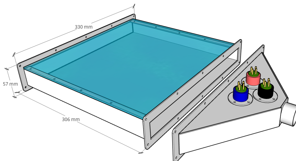
Rys. 1. Schemat poglądowy pojedynczego modułu i dyfuzora.
